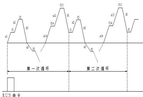
图 FC-1 PLC 单循环后停机示意图
