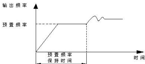
图 FA-4 闭环预置频率运行示意图
