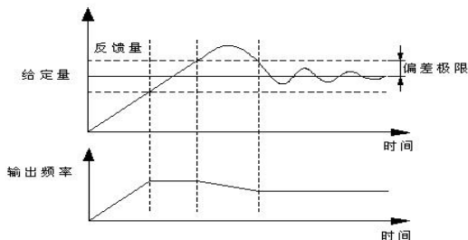
图 FA-3 偏差极限示意图
