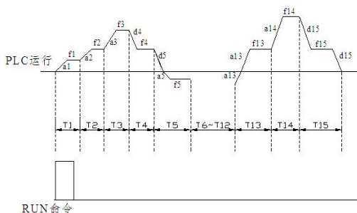
图 FC-2 PLC 单循环后保持示意图
