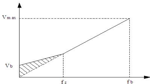
V_b -手动转矩提升量, f_z -转矩提升截止频率
